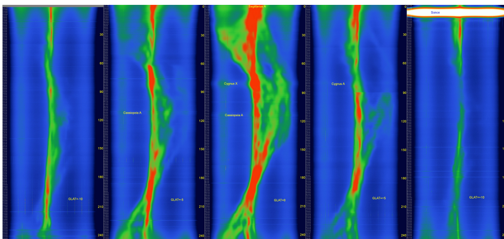
Slika 4.9: Spekter vodikove črte v naši Galaksiji pri različnih galaktičnih širinah
