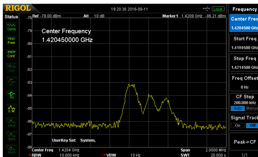
Slika 4.1: Meritev frekvenčnega spektra v smeri zvezde Deneba
