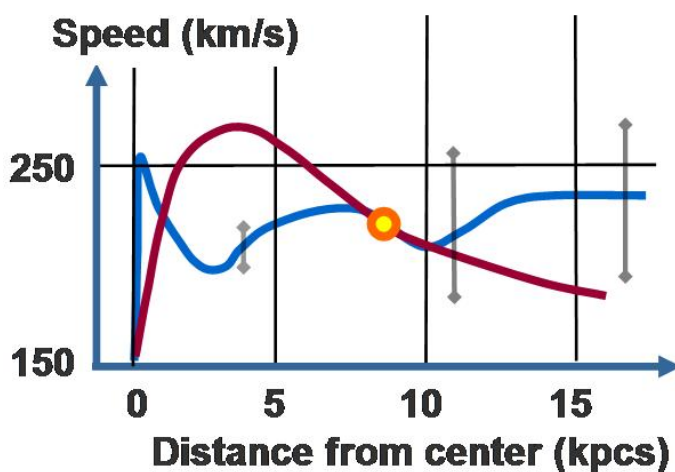
Slika 4.10: Izmerjena ter izračunana hitrost kroženja snovi v Galaksiji v odvisnosti od razdalje od središča [31]
