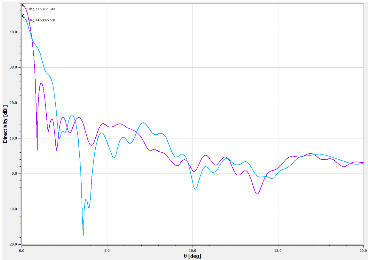
Slika 3 - 3.5m antenna
