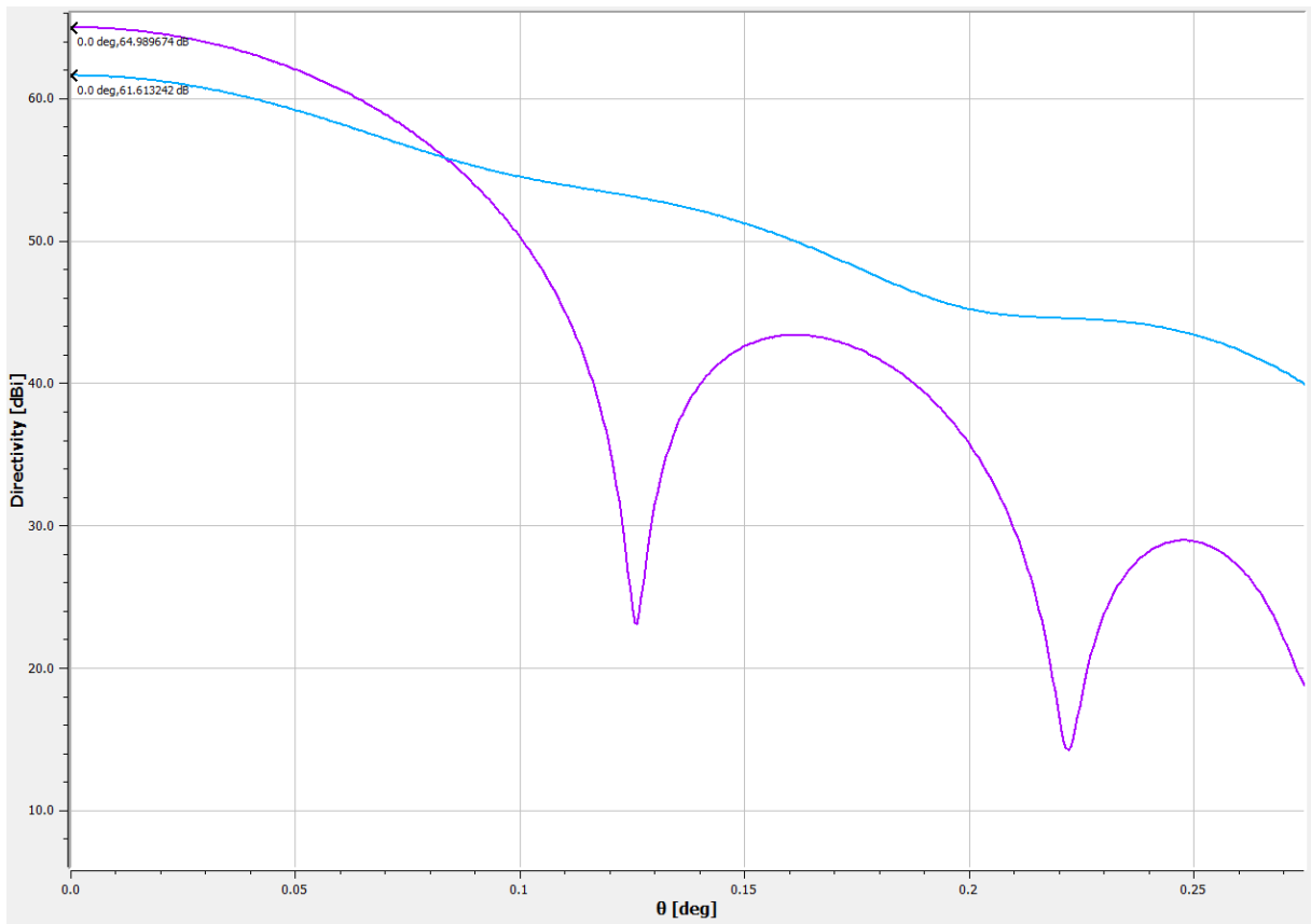
Slika 10 - 24m antena
