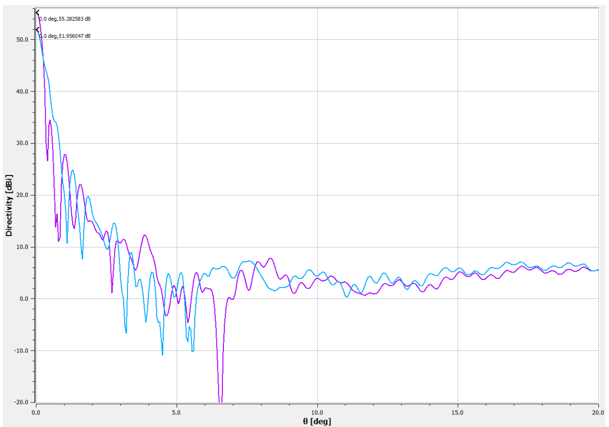
Slika 7 - 8m antenna
