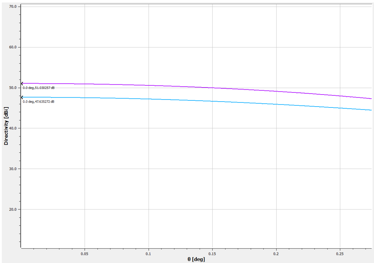
Slika 6 - 5m antenna
