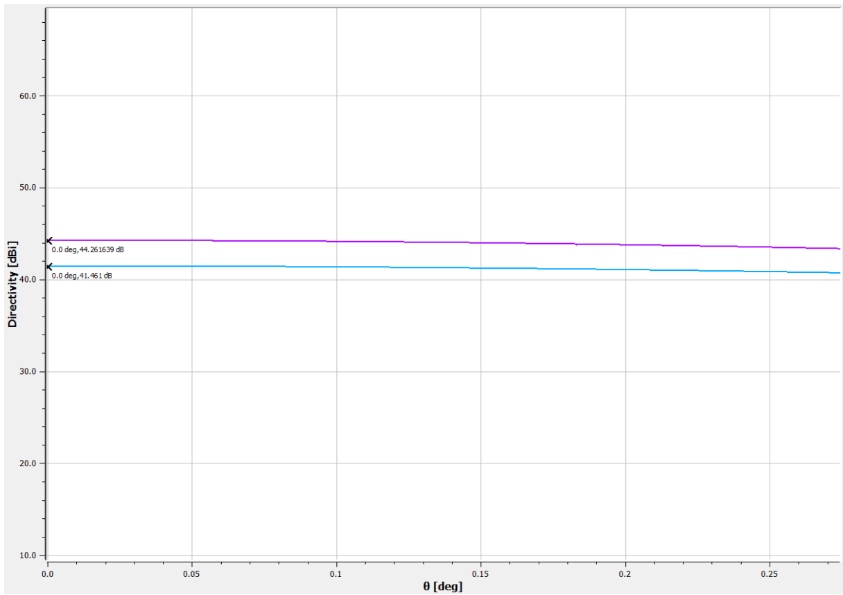
Slika 2 - 2.5m antenna
