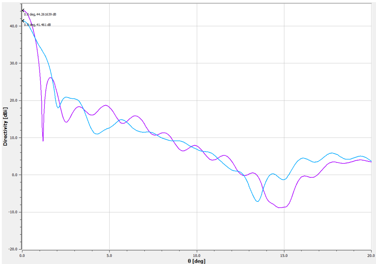
Slika 1 - 2.5m antena
