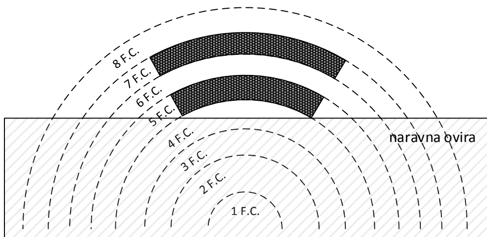
Slika 4: Difraktor iz delov con - trakov
