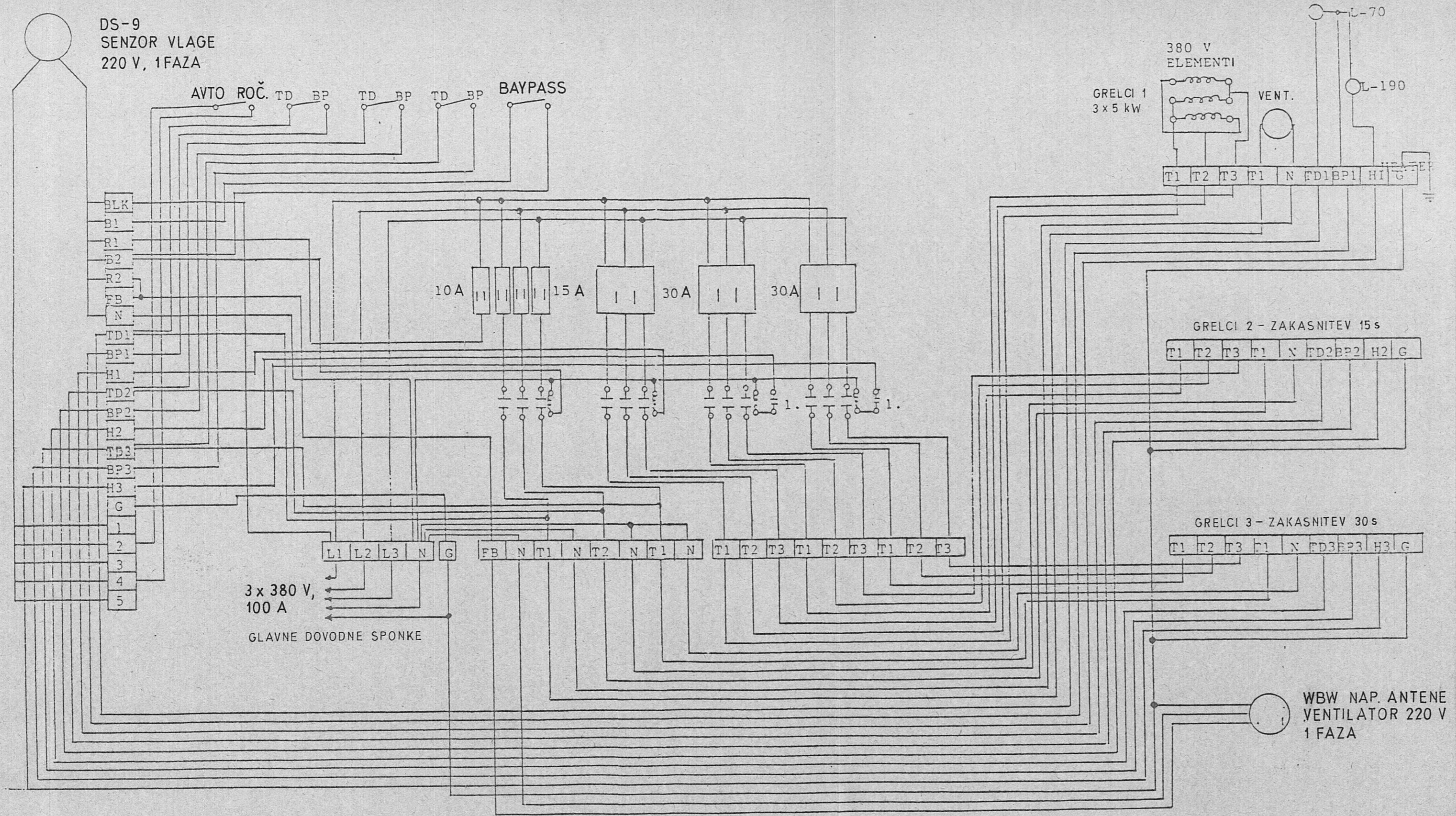
SISTEM ZA RAZLEDENITEV 3 x 15 kW IN ENOFAZNI VENTILATORJI
