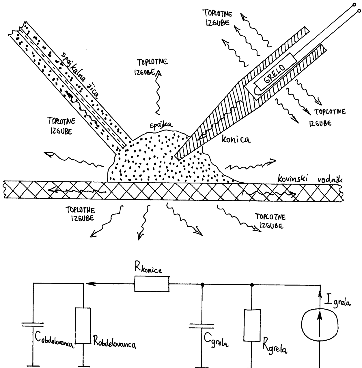
Slika 2 - Prenos toplote na mesto spajkanja
