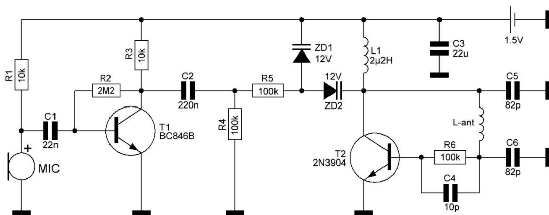
Slika 1: Shema FM radijskega oddajnika
