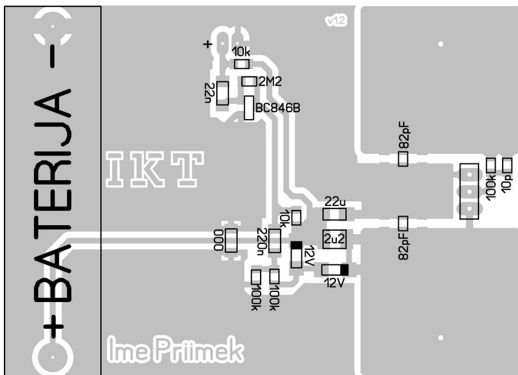
Slika 2: Postavitev elementov spodnja stran SMD
