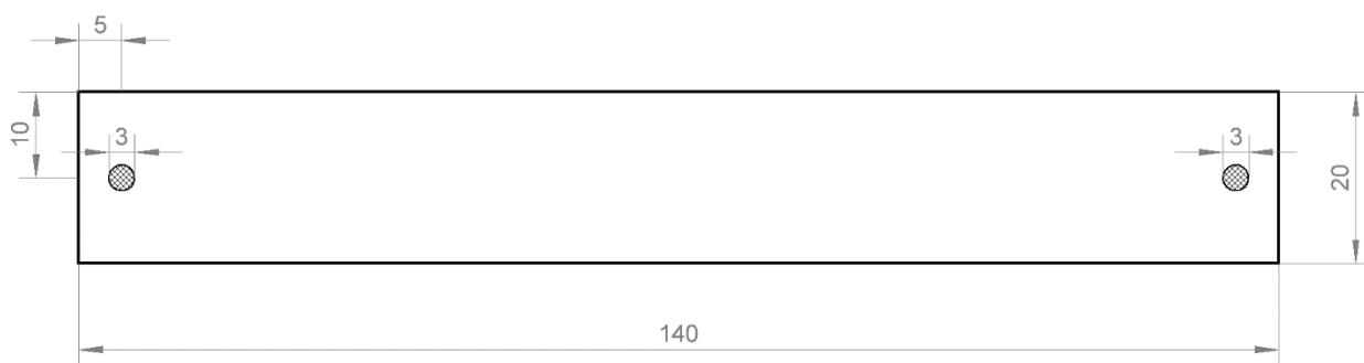
Slika 3: ALU trak kot oddajna antena
