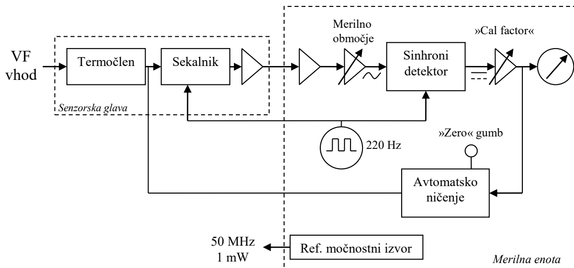
Slika 3: Poenostavljen blokovni načrt merilnika moči s termočleno senzorsko glavo.
