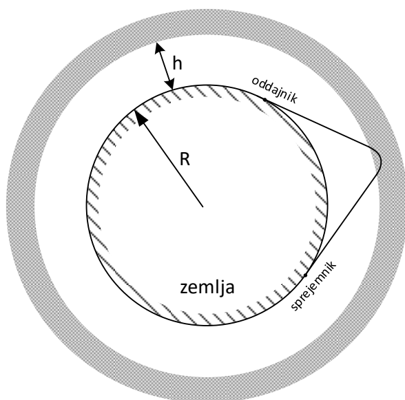
Slika 2: Najvišja frekvenca popolnega odboja (MUF).
