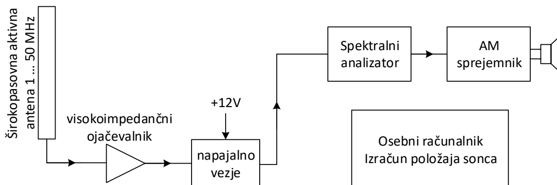
Slika 2: Skica vezave merilnih pripomočkov
