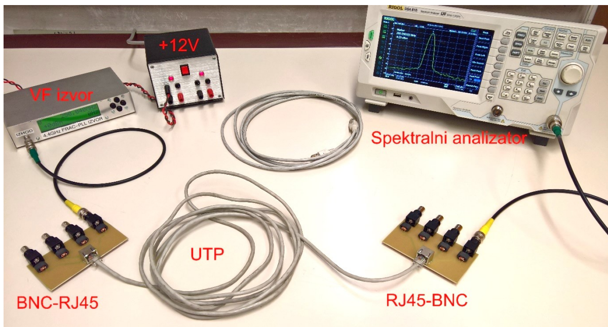
Slika 3: Slika vezave merilnih pripomočkov
